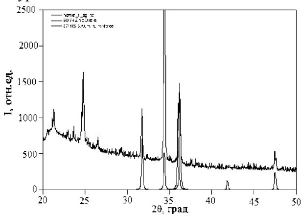
Рис. 4. Дифрактограмма пленки оксида цинка, полученной при температуре 773 К.
