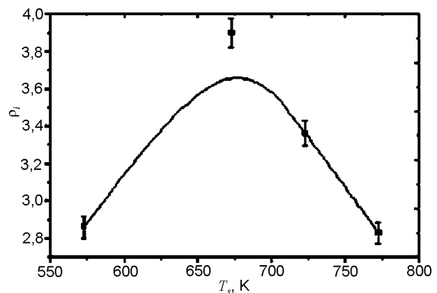
Рис. 5. Температурная зависимость полюсной плотности пленок оксида цинка.
