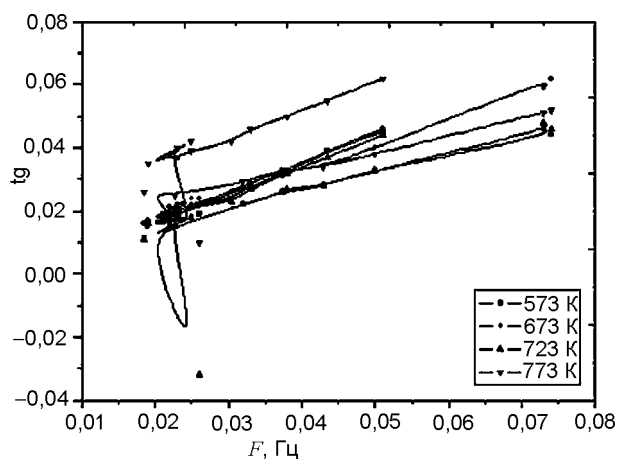
Рис. 7. Зависимость тангенса диэлектрических потерь пленок оксида цинка от частоты.
