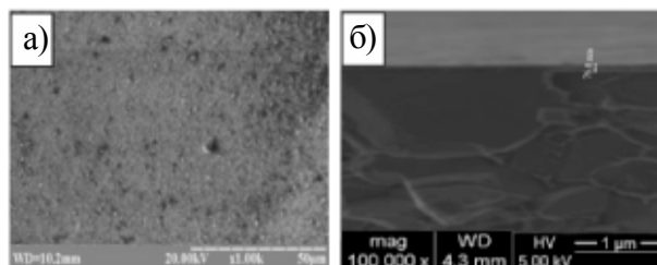
Рис. 2. Фрактограмма пленки AlN, полученного на подложке из стекла и морфология поверхности покрытия нитрида алюминия на кремнии: а) – в режиме контрастности (фазовый состав).
