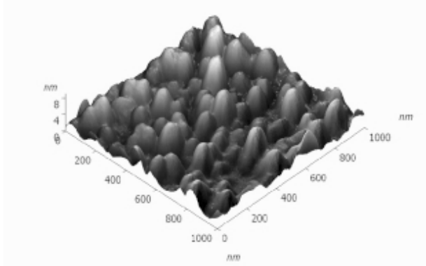
Рис. 3. Топография поверхности покрытия нитрида алюминия на кремнии, полученная с использованием сканирующего зондового микроскопа NTEGRA Aura в 3D формате.
