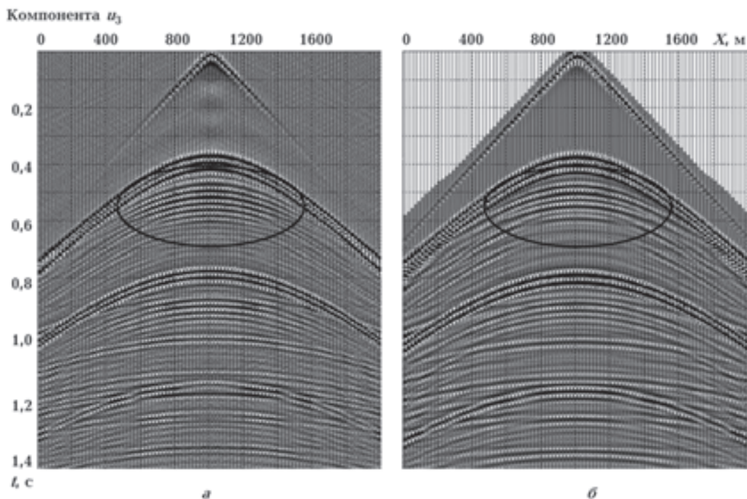
Рис. 6. Компонента u_3 зарегистрированного волнового поля, рассчитанная по методу Хаскелла—Томсона (а) и конечно-разностным методом (б). Овалами отмечены для сравнения отраженные волны от верхней части тонкослойистой пачки твердых слоев
