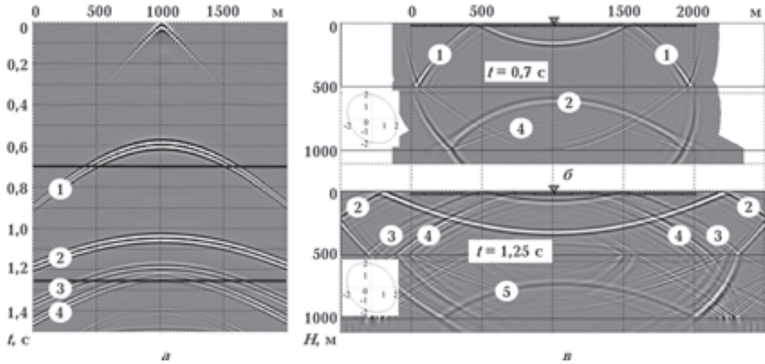
Рис. 4. u_3 -компонента волнового поля для трехслойной среды (а), зарегистрированная приемниками; срезы волнового поля (б, в) на временах t=0,7 с и t=1,25 с соответственно. Цифрами 1—5 обозначены разные типы волн, возникающих в процессе распространения.
