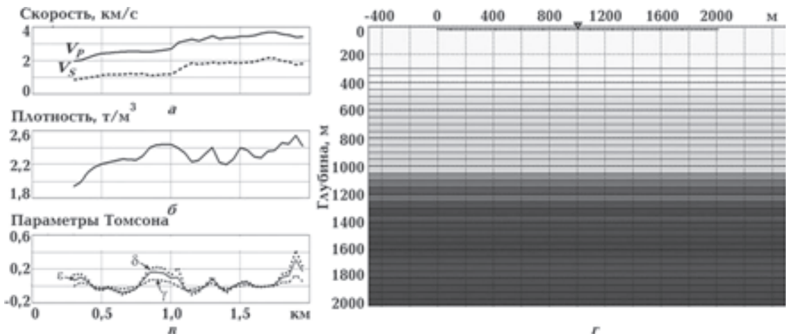
Рис. 5. Модель многослойной жидко-упругой среды с ВТИ-анизотропией, построенная по каротажным диаграммам для континентального шельфа Северного моря: а — кривые скоростей qP - и qSV -волн; б — кривые плотностей \rho ; в — кривые параметров Томсона \epsilon , \delta , \gamma ; г — вертикальное сечение среды и схема наблюдений.
