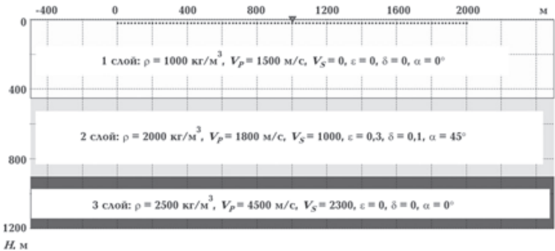
Рис. 3. Схема наблюдений и модель трехслойной среды, первый слой которой состоит из жидкости, второй — из твердой породы с ГТИ-анизотропией, третий — из твердой изотропной породы.
