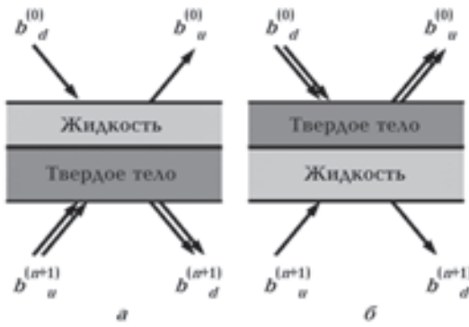
Рис. 2. Типы волн, возникающих при рассеянии на интерфейсе жидкость — анизотропная упругая среда: a — жидкость сверху, твердая порода снизу; b — жидкость снизу, твердая порода сверху.
