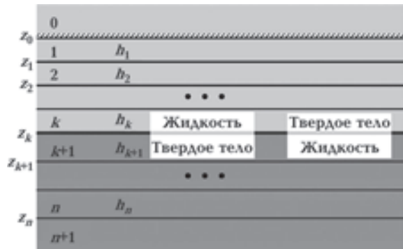
Рис. 1. Горизонтально-слоистая среда, состоящая из жидких и твердых анизотропных слоев.
