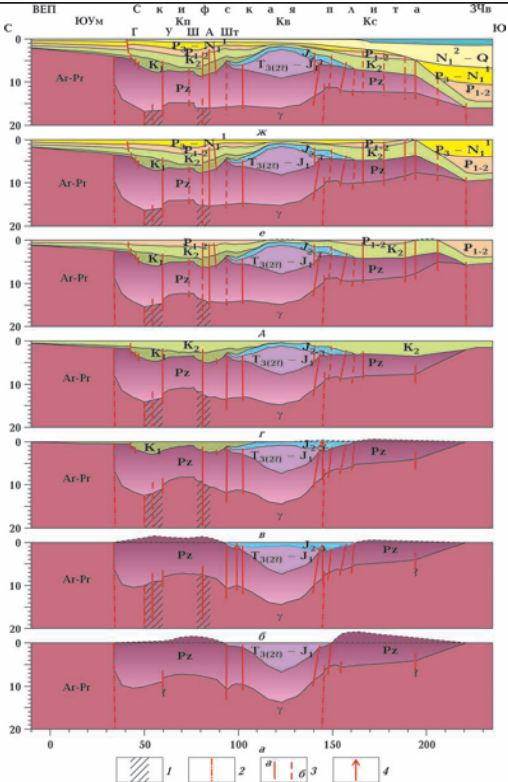
Рис. 3. Палеоструктурный разрез, построенный по данным МОВ ОГТ [Безверхов, 1988]. Обозначение структур см. рис. 2. Строение земной коры на момент: а — конец лейаса ( J_1 ); б — конец юры ( J_2 ); в — конец раннего мела ( K_1 ); г — конец позднего мела ( K_2 ); д — конец эоцена ( P_2 ); е — конец майкопа ( N_1^1 ); ж — современная структура ( Q ); 1 — высокоплотные блоки, выделенные по результатам гравитационного моделирования; 2 — транскорвые разломы по результатам плотностного моделирования; 3 — разломы по данным палеоструктурного профилирования (а — активные, б — «залеченные»); 4 — направление поступления вулканического материала.
