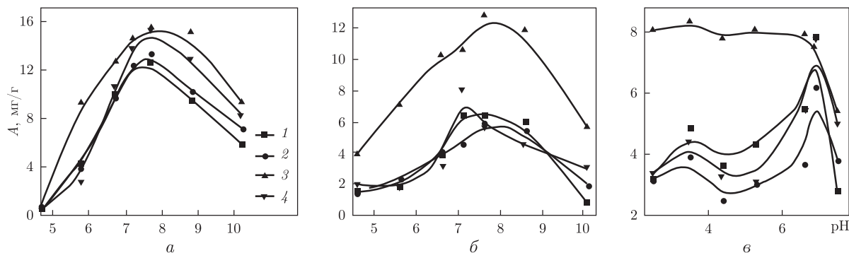
Рис. 1. Залежність адсорбції катіонів Zn^{2+} (а), Cd^{2+} (б) та Pb^{2+} (в) на поверхні синтезованих композитів від рН: 1 – Fe_3O_4 ; 2 – Fe_3O_4/SiO_2 ; 3 – Fe_3O_4/TiO_2 ; 4 – Fe_3O_4/Al_2O_3
