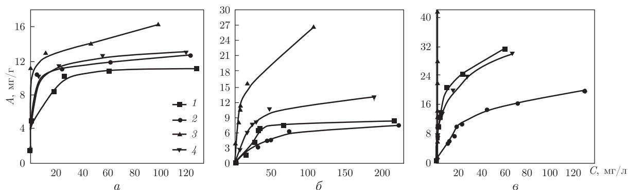
Рис. 2. Ізотерми адсорбції катіонів Zn^{2+} , рН 7,4 (а), Cd^{2+} , рН 7,54 (б) та Pb^{2+} , рН 7,0 (в) на поверхні композитів: 1 – Fe_3O_4 ; 2 – Fe_3O_4/SiO_2 ; 3 – Fe_3O_4/TiO_2 ; 4 – Fe_3O_4/Al_2O_3
