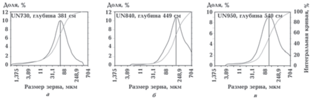
Рис. 7. Гранулометрический состав отложений горизонта ископаемой почвы P2 (а), песчаных горизонтов S5 (б) и S6 (в).
