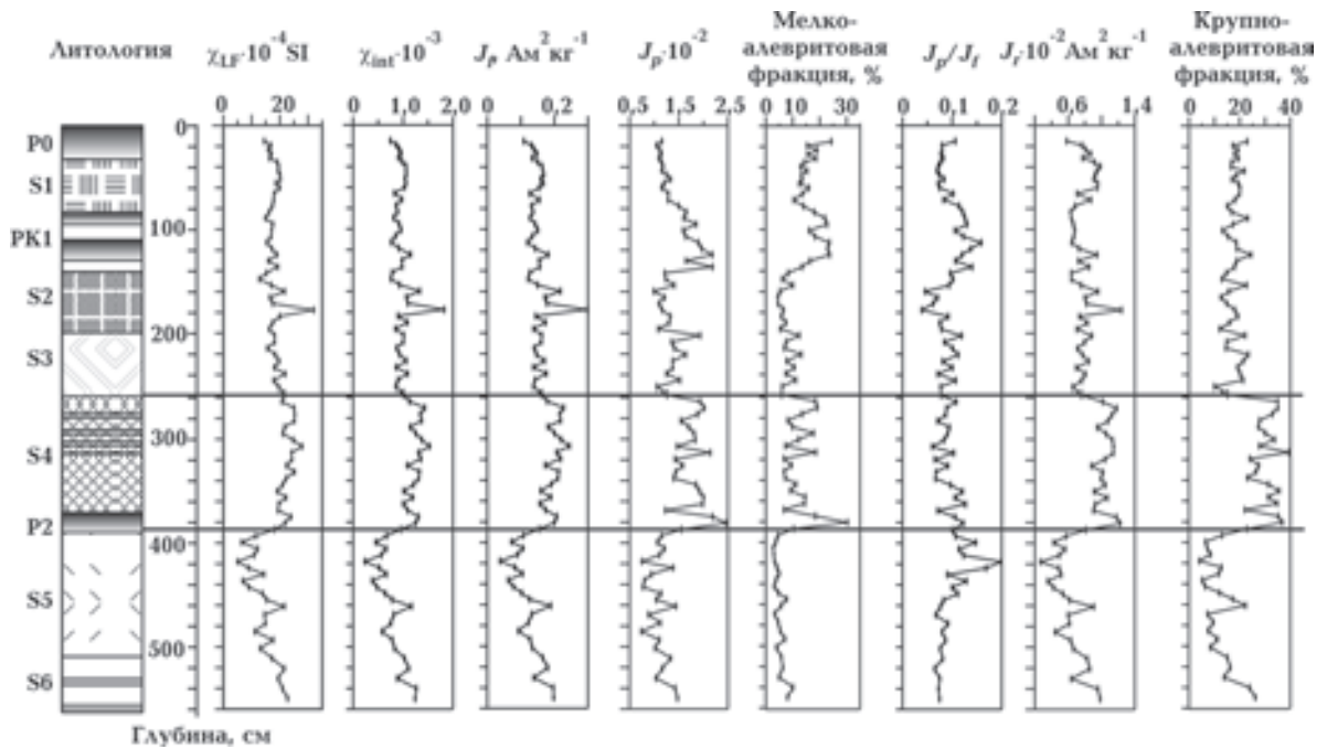
Рис. 8. Изменение концентрационно-зависимых параметров отложений по глубине: \chi_{LF} — низкочастотная магнитная восприимчивость; \chi_{int} — начальная магнитная восприимчивость; J_p — намагниченность насыщения ферромагнетиков, J_p — намагниченность парамагнетиков в поле 700 мТл; J_r — остаточная намагниченность.
