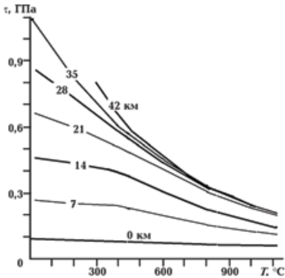
Рис. 3. Зависимость мгновенной прочности на сдвиг от температуры и давления (глубины) [Крылов, Дучков, 1996; Справочник ..., 1969, Петрофизика, 1992; Физические ..., 1988].
