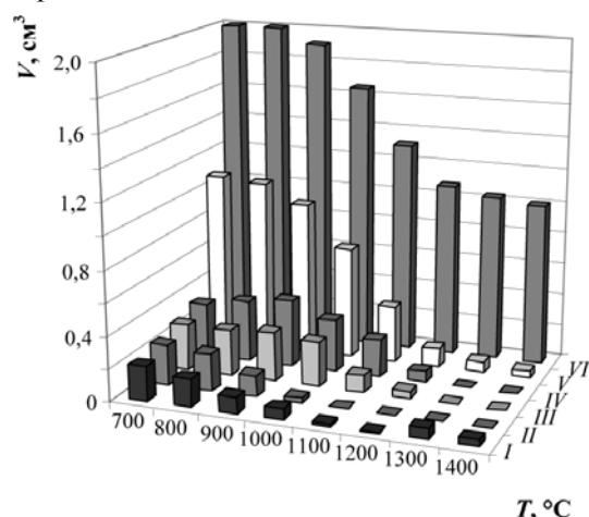
Рис. 2. Зависимости объемов поровых каналов и закрытых пор в пористых объектах из наноразмерного порошка кубического твердого раствора оксида циркония от температуры термообработки (выдержка 1 ч): I — закрытые поры; II — малые, III — средние и IV — большие поровые каналы; V — поровое пространство (все каналы и закрытые поры); VI — суммарный объем (объемы твердой фазы и порового пространства)
