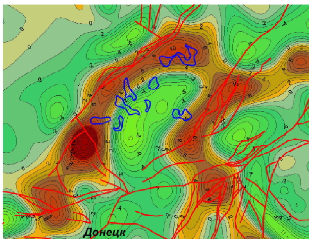
Рис. 2. Схема сопоставления прогнозных зон скопления метана в пределах поля шахты им. А.Ф. Засядько с напряжениями, обусловленными нарушением равновесного состояния [13]: а – скалывающие напряжения; б – напряжения сжатия–растяжения; 1 – тектонические нарушения; 2 – прогнозные зоны скопления метана
