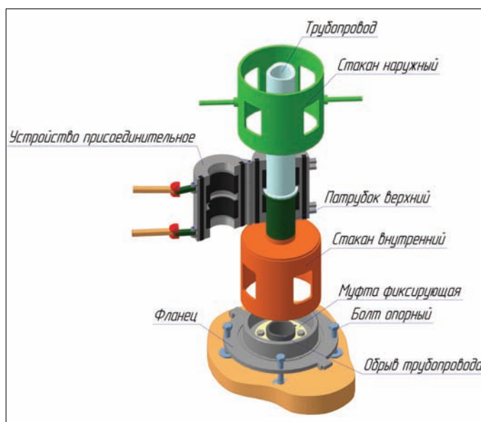
Модель аварийного модуля
