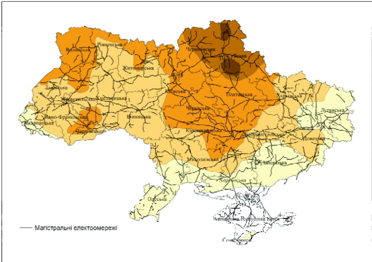
Рис. 4. Карта розташування магістральних електромереж в умовах загрози від танення снігу на території України. Умовні позначення див. на рис. 2
