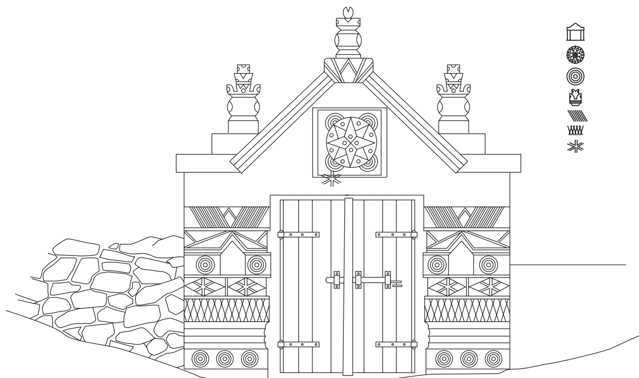
Портал пивниці в с. Желобок (Zhelobok), Орґеєвський р-н. (Будинок М. Блонтарь). Вирішений у вигляді двох пілонів перекритий трикутним фронтоном. Рисунок автора за матеріалами А. Захарова
