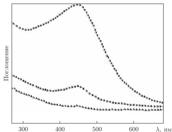
Рис. 1. Спектры поглощения в УФ и видимой области нанокмозитов ПУМ-НС 0,0016 (1), ПУМ-НС 0,016 (2) и ПУМ-НС 0,16 (3)
