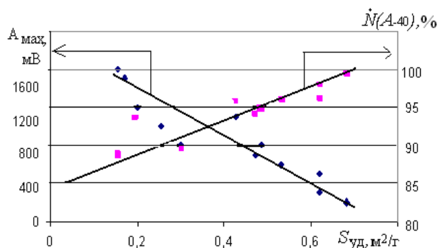
Рис. 2 – Зависимости величины максимальной амплитуды и доли малоамплитудных сигналов от удельной поверхности измельченных материалов плотностью 2,8 – 3,0 г/см 3
