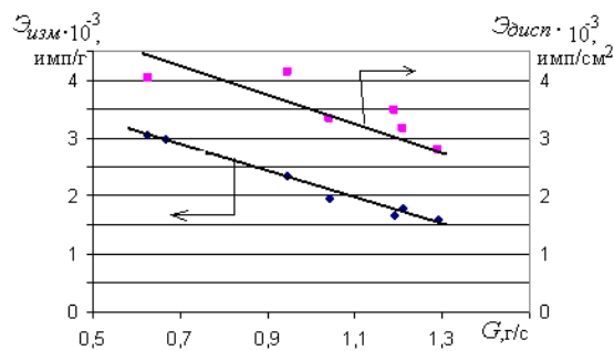
Рис. 4. – Зависимости показателей энергоёмкости измельчения \mathcal{E}_{изм} и диспергирования \mathcal{E}_{дисп} кварцевого песка от производительности лабораторной струйной мельницы УСИ-20 (при давлении энергоносителя P_0 = 0,3 МПа, оборотах классификатора n = 2500 - 3000 мин -1 , S_{уд} = 0,48 - 0,75 см 2 /г).
