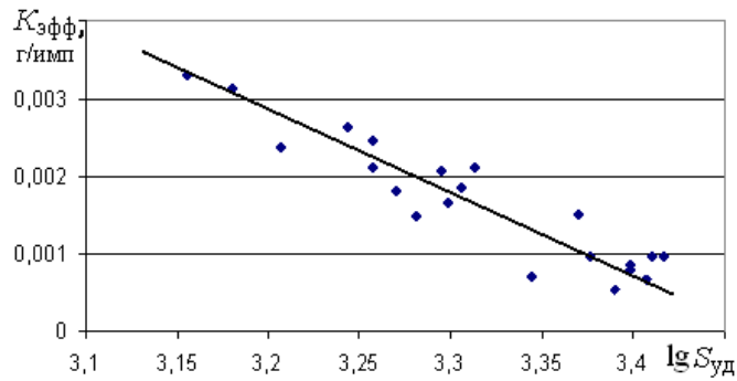
Рис. 3 – Зависимость коэффициента эффективности от удельной поверхности измельченных материалов
