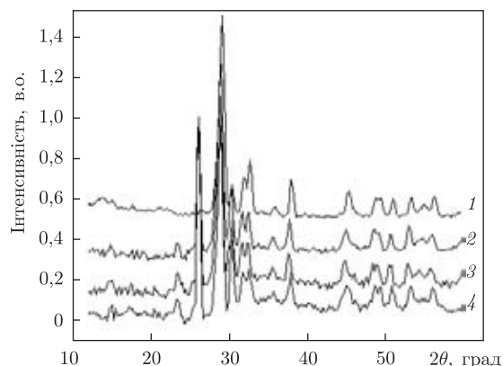
Рис. 2. Рентгенівські дифрактограми зразків: 1 – порошок РbО; 2 – ЕП-3%РbОпмп; 3 – ЕП-3%(РbО+ПАН) н.у.; 4 – ЕП-3%(РbО + ПАН)пеп
