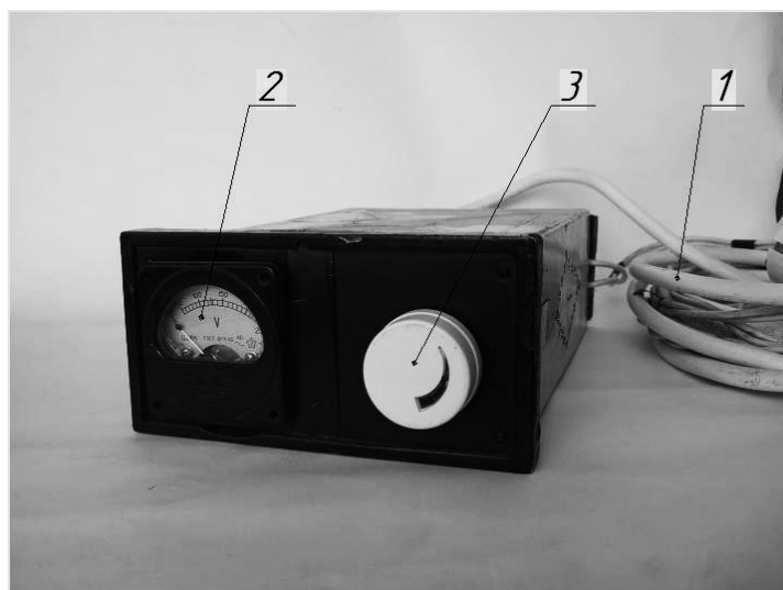
Рис. 3 – Общий вид блока управления нагревом выработки
