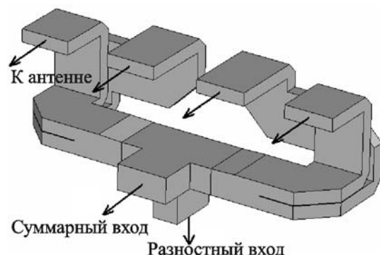
Рис. 8. Волноводный компаратор
