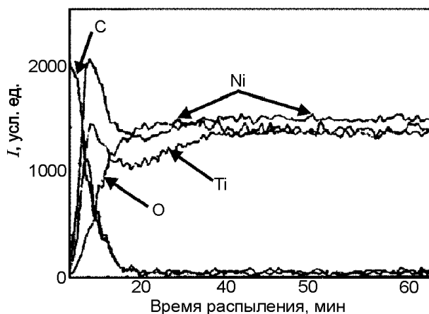
Рис. 4. Элементный состав (оже-профили), полученный с образцов сплава – TiNi, после имплантации азотом (энергия 60 кэВ, доза 10^{18} см -2 ).
