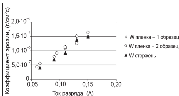
Рис. 6. Зависимость скорости эрозии от тока плазменного разряда.
