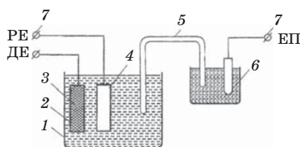
Рис. 1. Принципова схема устави для електрохімічних досліджень потенціостатичних та потенціодинамічних характеристик напівпровідників: 1 — поляризаційна комірка; 2 — розчин електроліту; 3 — допоміжна електрода (ДЕ); 4 — робоча електрода (РЕ); 5 — соляний місток; 6 — електрода порівняння (ЕП); 7 — відповідні клемми потенціостату Scanning Potentiostat mod. 362 EG&G PARC.
