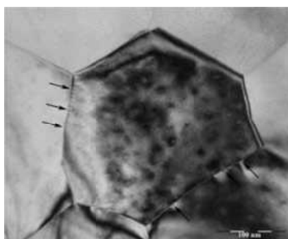
Рис. 2. Электронно-микроскопическое светлополюсное изображение тонкой структуры фольг Fe–W.
