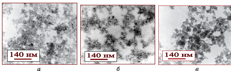
Рис. 2. Морфология модифицированных нанопорошков магнетита (водная среда): а — \text{NH}_2\text{CH}_2\text{COOH} ; б — \text{SHCH}_2\text{COOH} ; в — \text{CH}_3\text{CH}_2\text{COOH} .
