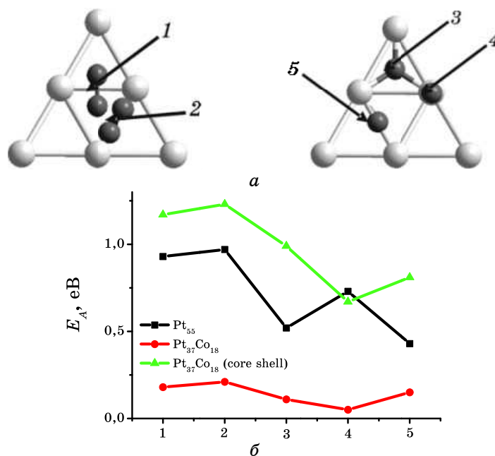
Рис. 2. Місця адсорбції (а) та розраховані енергії активації адсорбції (б) молекули кисню на поверхні (111) нанокластерів платини: 1 — чотирицентрове; 2 — двоцентрове; 3 — трицентрове; 4 — надатомове; 5 — місткове.
