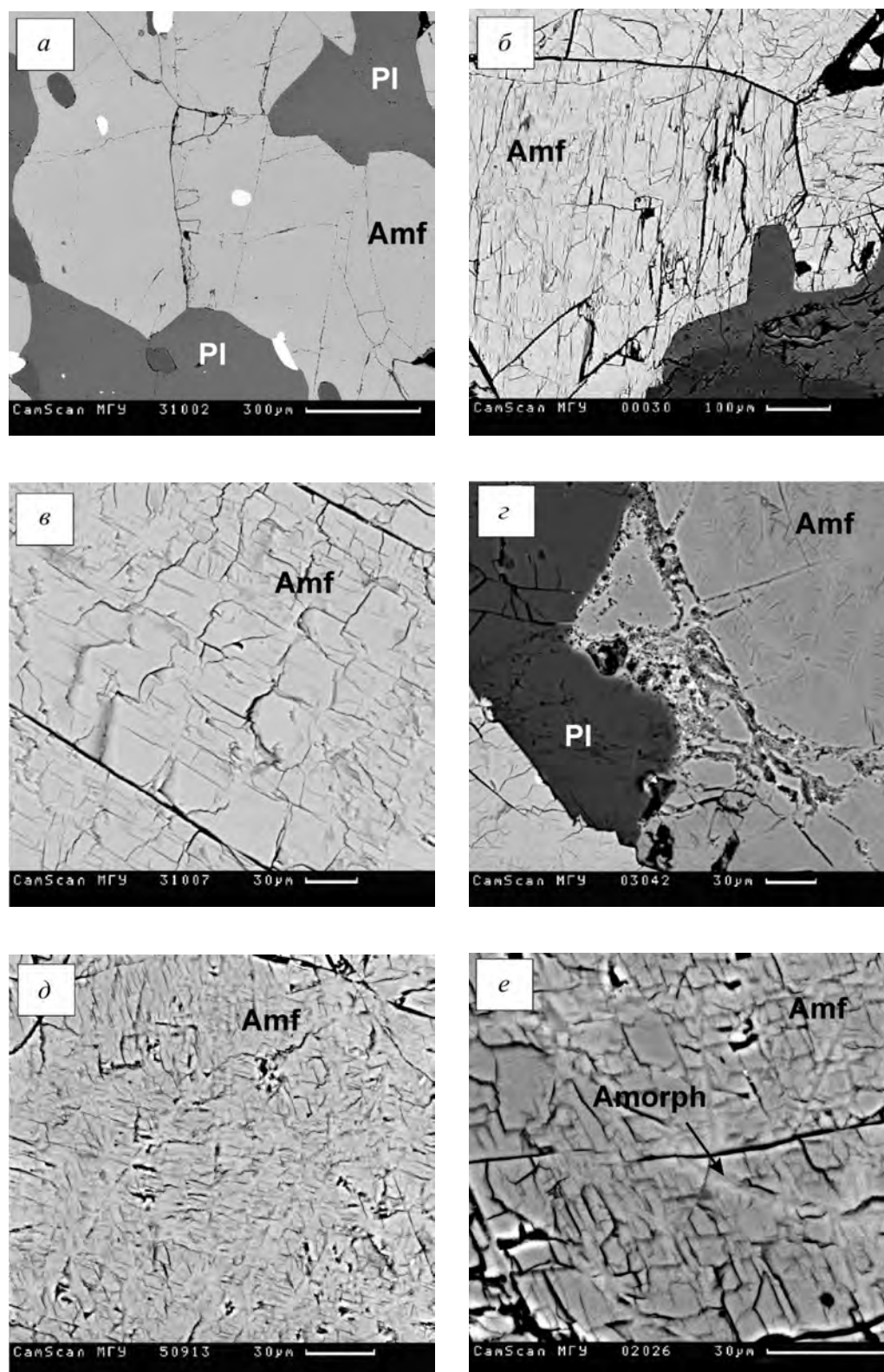
Рис. 4. Амфибол в образцах кристаллических сланцев: ДН-31/1: a – исходный; b , в , г – испытывавшие ударную нагрузку (GPa) соответственно 26, 36 и 52; 73-509а-1: д , е – испытывавшие нагрузку (GPa) соответственно 36 и 52
