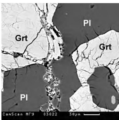
Рис. 2. Участки пористого материала в PI образца ДН-31/1, испытавшего ударную нагрузку 52 GPa
