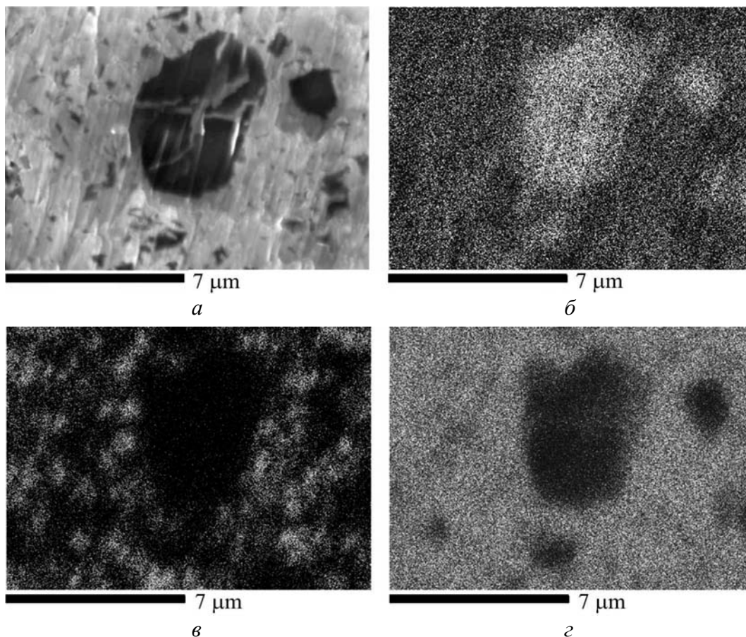
Рис. 3. Данные обратного рассеяния электронов и анализ распределения элементов образцов на основе MgB_2 из Mg и B(III) с 10 mass% Ti, взятых в отношении 1:2, синтезированных при 2 ГПа и температуре 1050°C в течение 1 h: a – электронное изображение; б , в , г – распределение соответственно бора, кислорода и магния. Более светлые области соответствуют большему количеству исследуемого элемента
