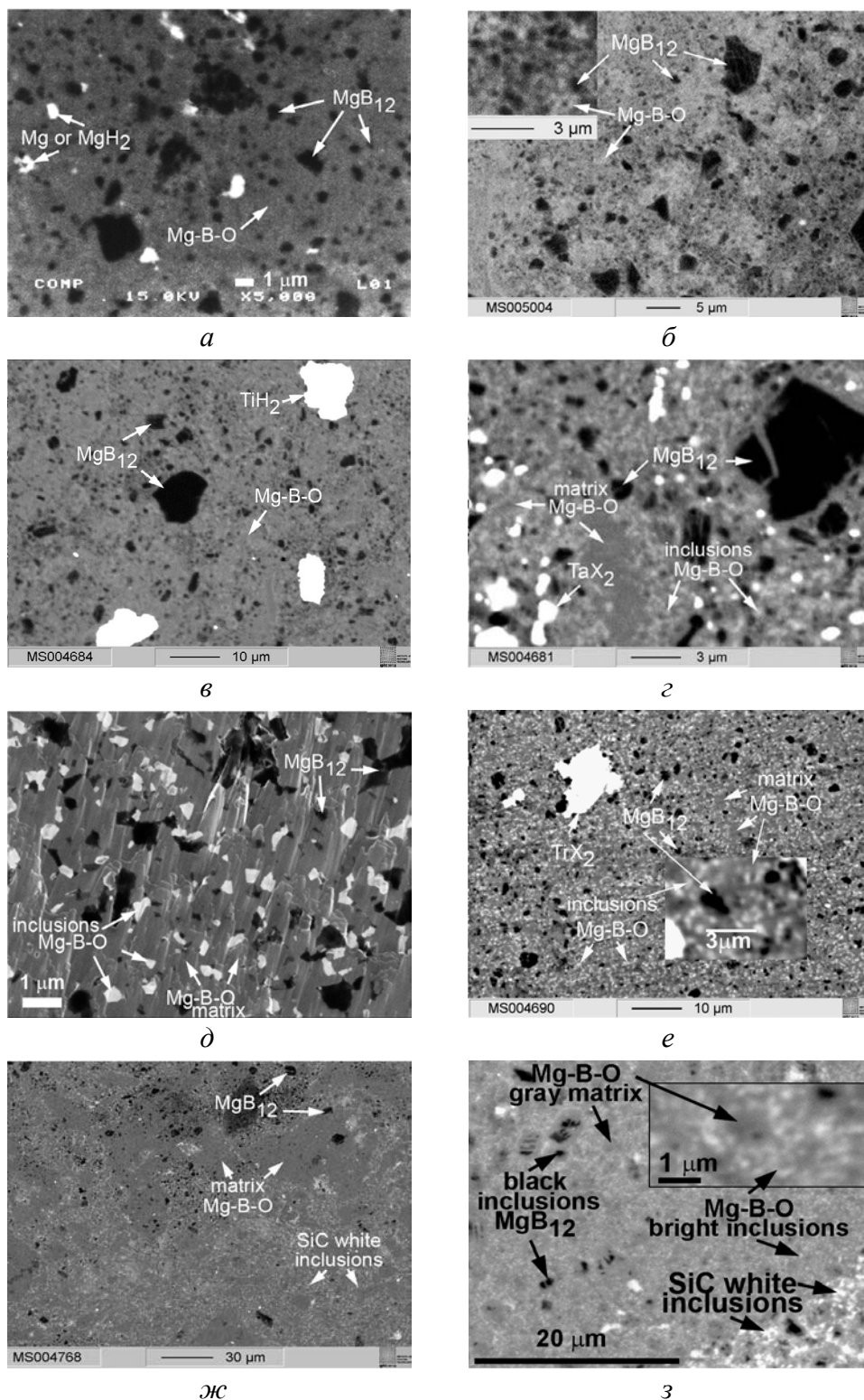
Рис. 2. Данные обратного рассеяния электронов микроструктур на основе MgB_2 , синтезированных из Mg и B, взятых в отношении 1:2 при 2 GPa в течение 1 h: a, б – из B(III) соответственно при 800 и 1050°C; в – из B(III) с 10 mass% Ti при 800°C; г – из B(III) с 10 mass% Ta при 1050°C; д, е – из B(III) с 10 mass% Ti при 1050°C при различных увеличениях; ж, з – из B(I) с 10 mass% SiC при 1050°C при различных увеличениях
