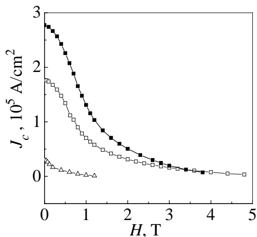
Рис. 4. Зависимости плотности критического тока от величины магнитного поля для исследованных образцов при T = 15 К: \square – MgB_2 + SiC , \triangle – MgB_2 , \blacksquare – MgB_2 + TiO_2
