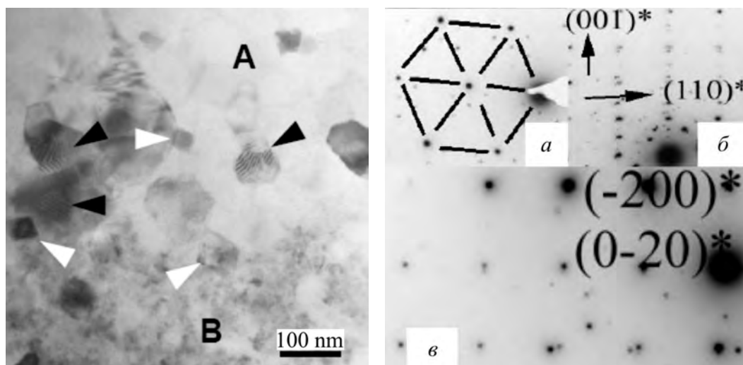
Рис. 2. Снимок ТЕМ высокого разрешения для \text{MgB}_2 + \text{TiO}_2 . А и В обозначают области крупно- и мелкозернистой микроструктур соответственно. Черные стрелки – муаровые интерференционные полосы, белые – включения \text{MgO}
