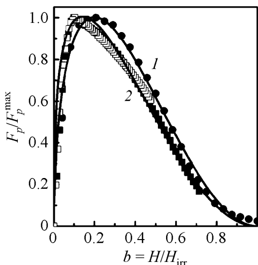
Рис. 7. Магнитно-полевые зависимости приведенной плотности силы пиннинга для образца \text{MgB}_2 + \text{SiC} при 5 ( -\square- ), 15 ( -\blacksquare- ) и 25 ( -\bullet- ) К: 1 – b^{0.5}(1-b)^2 , 2 – b^{0.3}(1-b)^2
