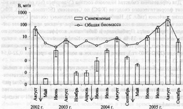
Рис. 1. Межгодовая и сезонная динамика биомассы синезелёных водорослей и общей биомассы фитопланктона в Берешском водохранилище.
