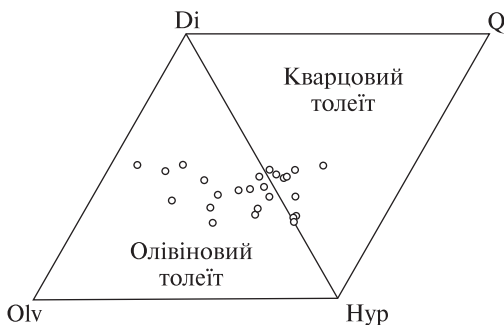
Рис. 9. Класифікація базитів за нормативним складом (Thompson, 1984). Коломи позначений нормативний склад лейкократових амфіболітів
