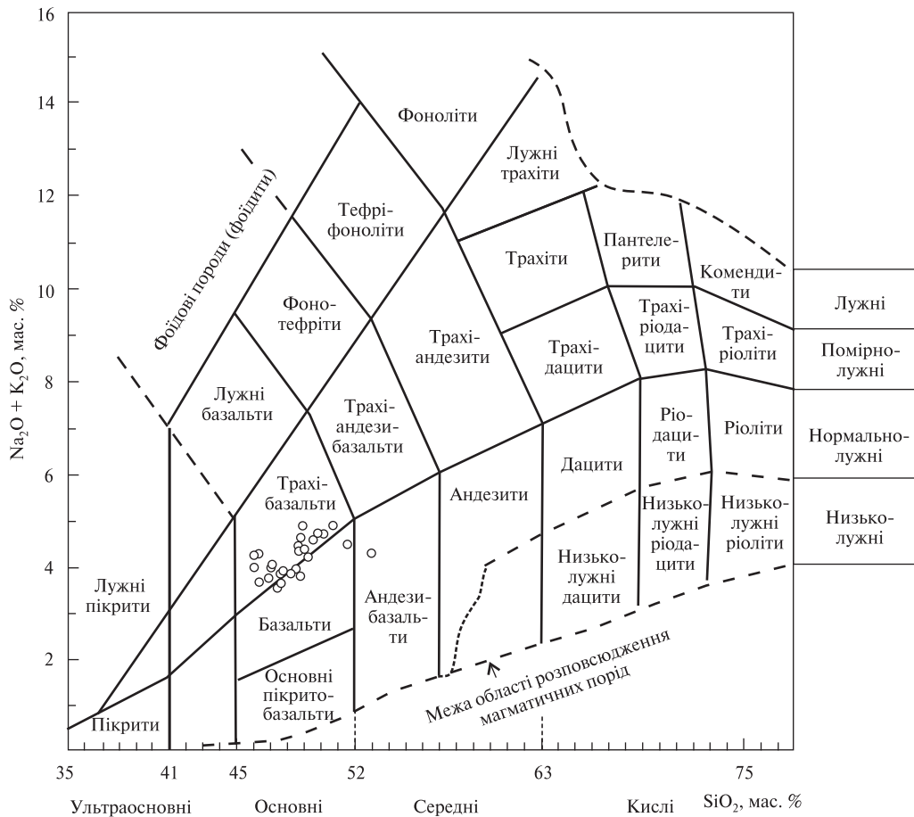
Рис. 6. Положення лейкократових амфіболітів на діаграмі TAS Fig. 6. Leucocratic amphibolites' position in TAS diagram
