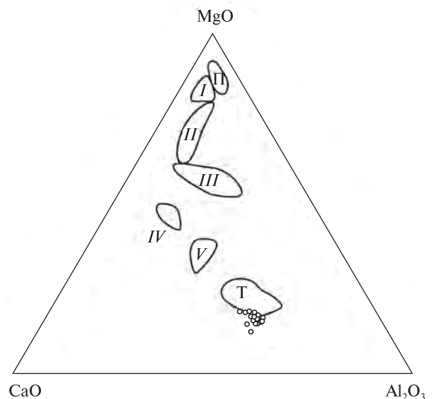
Рис. 10. Поля кристалізації лейкократових амфіболітів, за М.І. Viljoen, Р.Р. Viljoen. П — перidotитові коматити, Т — толейтові базальти
