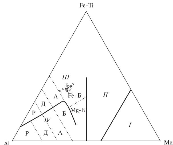
Рис. 11. Класифікаційна діаграма Al - (Fe + Ti) - Mg (Jensen, Pyke, 1982): I — коматіти, II — коматітові базальти, III — вулканіти толеїтової та IV — вапнисто-лужної серій; P — ріоліти, Д — дацити, А — андезити, Б — базальти. Поля базальтів: Mg-Б — високомагнієвих базальтів; Fe-Б — високозалізистих толеїтової серії. Колами позначений склад лейкократових амфіболітів
