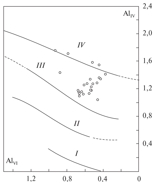
Рис. 5. Положення рогових обманок із лейкократових амфіболітів на діаграмі розподілу Al_{IV} - Al_{VI} . Фації метаморфізму: I — зеленосланцева, II — епідот-амфіболітова, III — амфіболітова, IV — гранулітова
