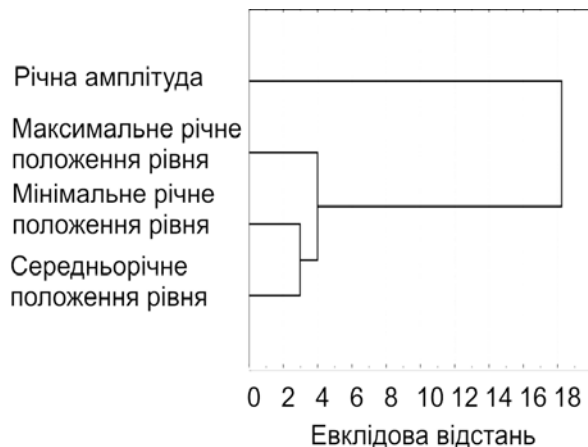
Рис. 5. Дендрограма зв'язків між параметрами багаторічного рівневого режиму для свердловини № 242004355
