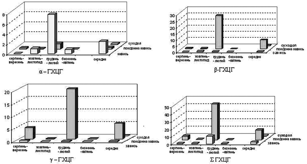
Рис. 3. Розподіл ГХЦГ та його ізомерів у складі завислої речовини в різні сезони, \text{mg/kg} \cdot 10^{-3}
