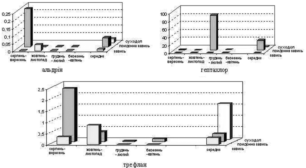
Рис. 4. Розподіл альдрину, гептахлору, трєфлану у складі завислої речовини в різні сезони, \text{mg/kg} \cdot 10^{-3}
