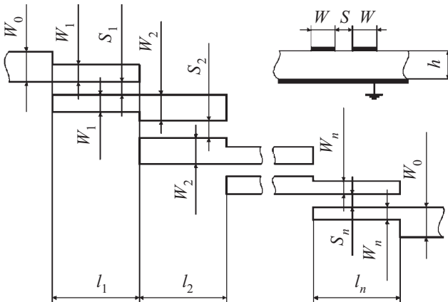
Рис. 1. Топология фильтра на связанных линиях: W_i — ширина связанных линий фильтра; S_i — зазоры между связанными линиями; l_i — длина звеньев фильтра; h — толщина диэлектрической подложки
