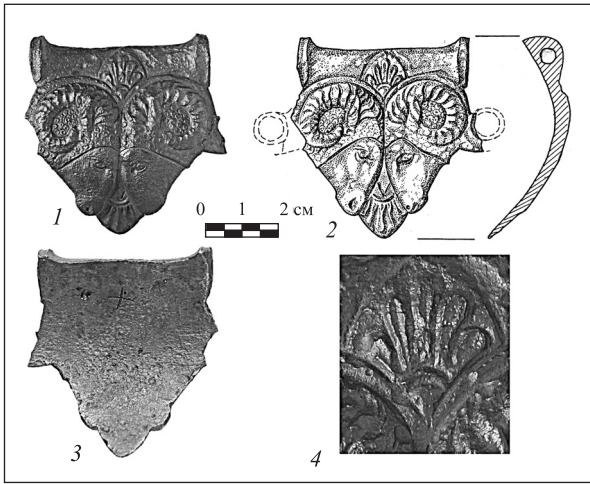
Рис. 4. Агташ ручки бронзового таза зі Східної могили Бердянського кургану: 1 — лицьовий бік (фото); 2 — лицьовий бік та перетин (рисунок); 3 — зворотний бік із хрестоподібною міткою; 4 — розетка
