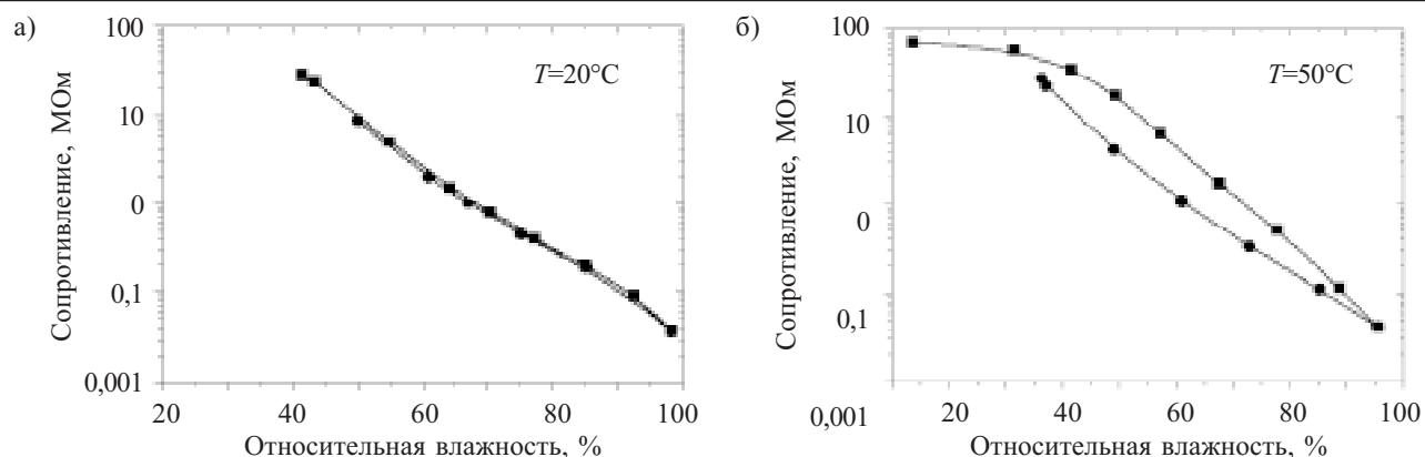
Рис. 1. Типичные эксплуатационные характеристики влажочувствительности толстых пленок MgAl 2 O 4 при температуре 20 (а) и 50°C (б), полученные при увеличении (■) и уменьшении (●) относительной влажности
