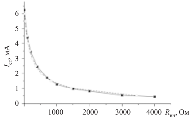
Рис. 3. Экспериментальные (■) и расчетные (○) данные зависимости тока стабилизации от R_{вн}
