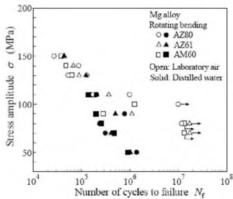
Fig. 1. S-N diagram.
