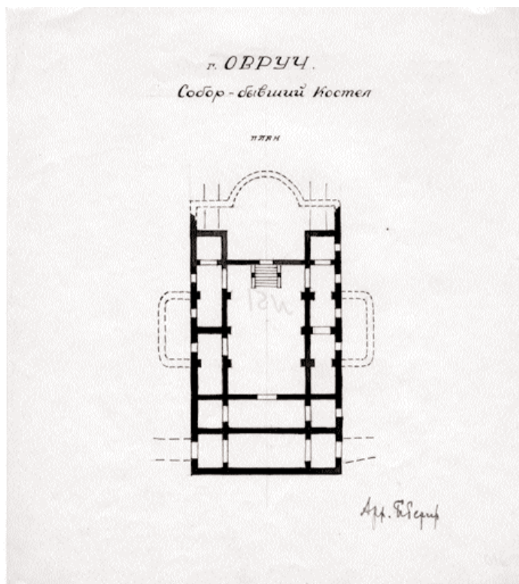
Овруч. Собор (колишній римо-католицький костел). Схема плану. 1909 р. Чорнило, папір. Ф. 14-9, од. зб. 662, арк. 12
