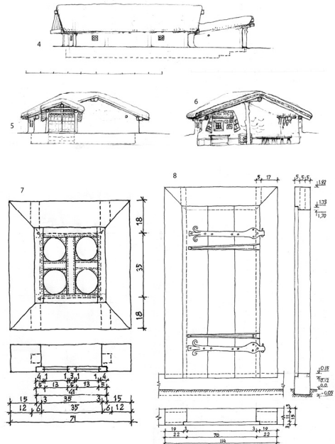
Табл.2. 4. Південний фасад; 5. Східний фасад; 6. Поперечний перетин; 7. Вікно; 8. Двері
