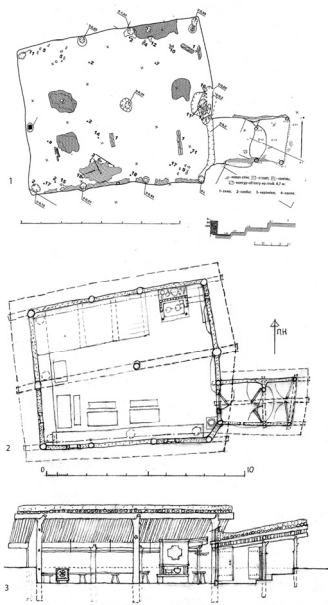
Табл.1. 1.План куреня за археологічними дослідженнями Козловського А.О. та Іллінського В.Є.; 2. План куреня за пропозиціями відтворення; 3. Поздовжній перетин
