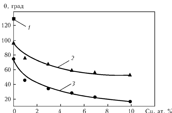
Рис. 1. Зависимость краевого угла смачивания \theta керамики \text{BaTiO}_3 расплавами системы \text{Ag-Cu-O} от содержания в них меди при 980 °С: 1 — расплав чистого серебра в вакууме; 2, 3 — расплав системы \text{Ag-Cu} соответственно в воздушной среде и чистом кислороде
