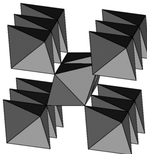
Fig. 2. Rutile structure
