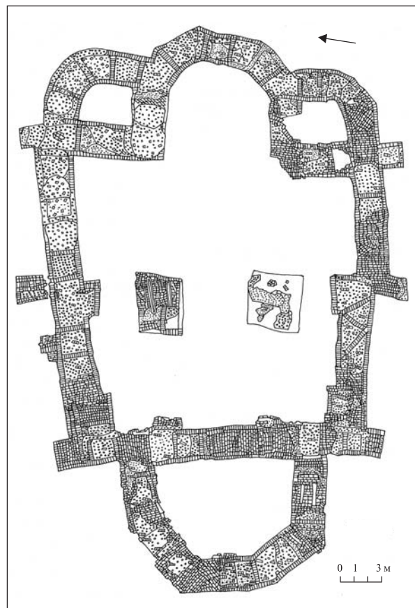
Рис. 2. Батурин. План фундаментів Церкви Живоначальної Трійці
