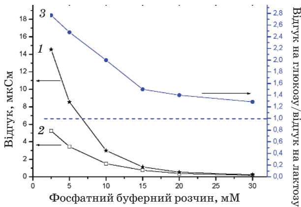
Рис. 6. Залежність величин відгуків біосенсора на 0,1 мМ глюкози (1) і 0,1 мМ лактози (2) та співвідношення відгуків на 0,1 мМ глюкози та 0,1 мМ лактози (3) від буферних розчинів різної концентрації
