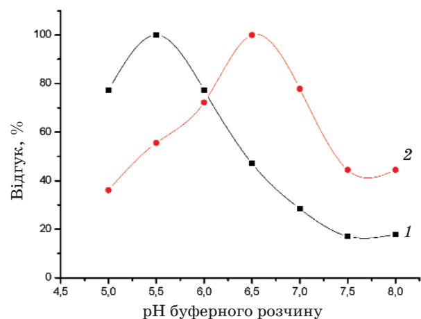
Рис. 8. Графік залежності відгуків лактозного біосенсора від рН розчину в разі додавання 0,5 мМ глюкози (1) та 0,5 мМ лактози (2). Вимірювання проводили в 10 мМ фосфатному буферному розчині. За 100% взято максимальну величину відгуків відповідного субстрату
