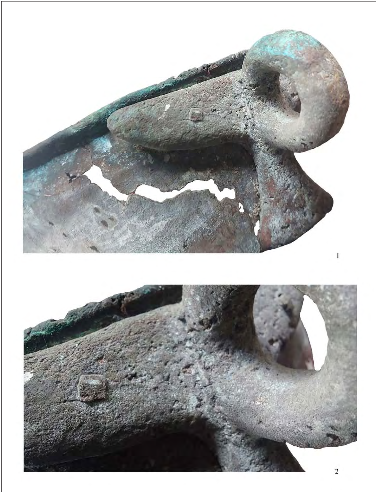
Рис. 10. Залишки зварювальних швів у місці з'єднання фігурної накладки з фіксованим кільцем на атташі з кургану Реп'яхувата Могила: 1 — загальний вигляд; 2 — збільшено. (Фото І. Б. Шрамко)
