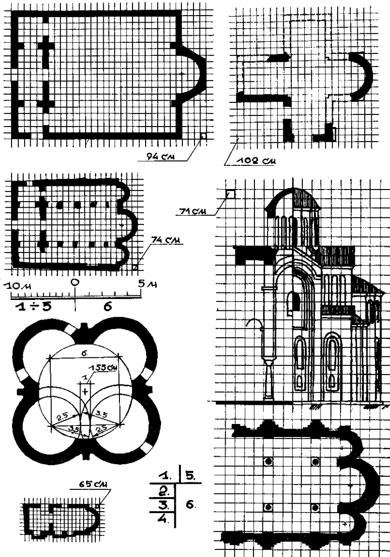
Рис. 3. Схеми модульної побудови: 1. Базиліка на Мангупі, 2. Парте́нітська базилика, 3. Чотириапсидний храм, 4. Храм з аркасоліями, 5. Храм під собором, 6. Церква Іоанна Предтечі (№ 3—5 знаходяться в Херсонесі).
