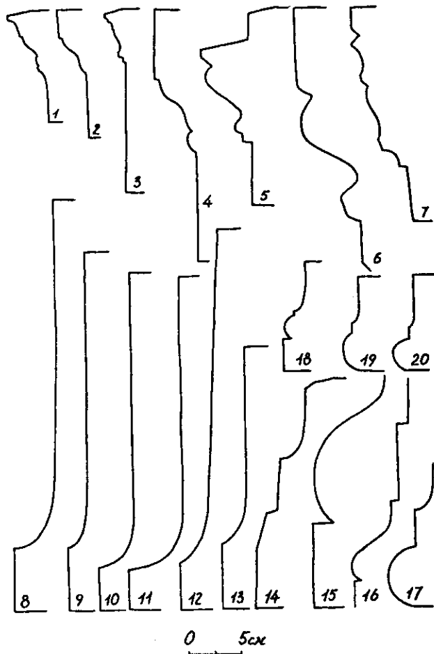
Рис. 4. Капітелі аттичного ордеру: 1, 2, 5 — Херсонес, 3 — Калос Лімен, 4 — Мірмекій, 6 — Ольвія, 7 — Танаїс. Бази аттичного ордеру: 8—13, 15—17 — Ольвія, 14 — Танаїс, 18 — Раєвське городище, 19, 20 — резиденція Хрисаліска (4 — за В. Ф. Гайдукевичем, 6, 16, 17 — за С. Д. Крижицьким, 18 — за Н. О. Онайко, 19, 20 — за М. І. Сокольським, 7, 14 — за Т. М. Арсеньєвою, Д. Б. Шеловим, в усіх інших випадках обміри виконані автором).
