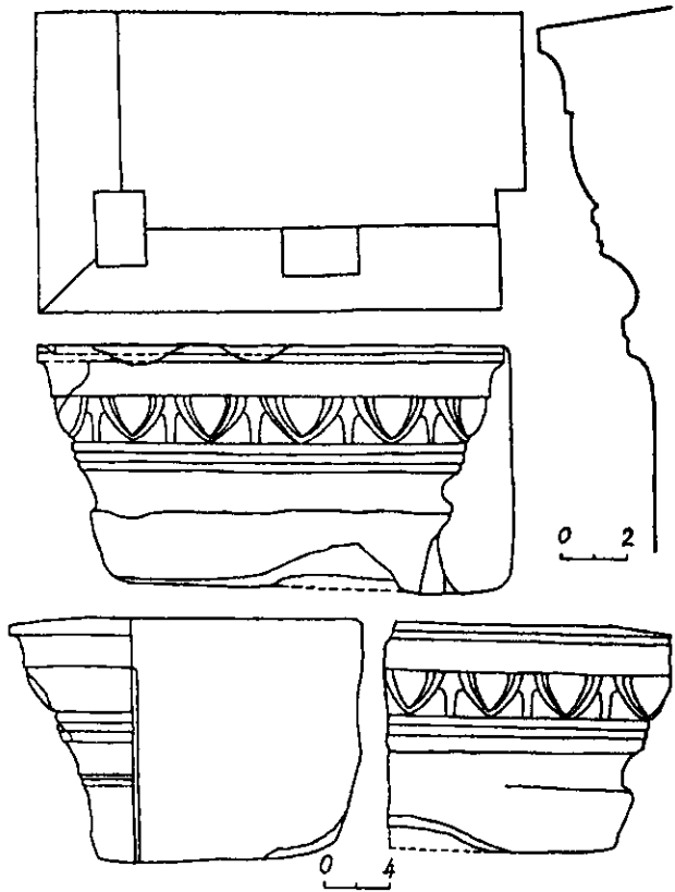
Рис. 2. Капітель аттичного ордеру з Ольвії.
