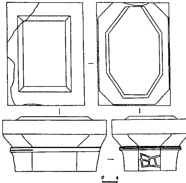
Рис. 3. Капітель аттичного ордера з Херсонеса.
