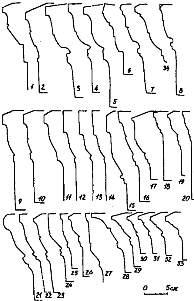
Рис. 1. Капітелі аттичного ордера: 1—7, 17, 18, 21—23, 27, 34 — Ольвія; 8, 11—14, 16, 19, 20, 24—26 — Херсонес; 9, 10 — городище «Чайка»; 28 — Раєвське городище; 29—33 — резиденція Хрисаліска. (1—5, 7, 21—23 — за С. Д. Крижицьким, 9, 10 — за І. В. Яценко, Т. М. Туриною, 28 — за Н. О. Онайко, 30—33 — за М. І. Сокольським, в усіх інших випадках обміри виконані автором).
