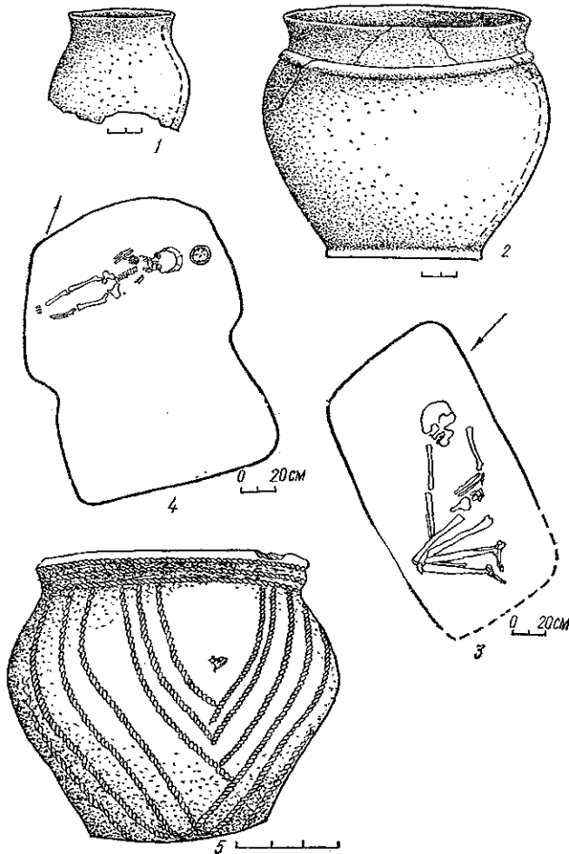
Ігреньський п-ів. Матеріали розкопок поселення епохи бронзи (1, 2) та поховань № 1 (3), 2 (4, 5).
