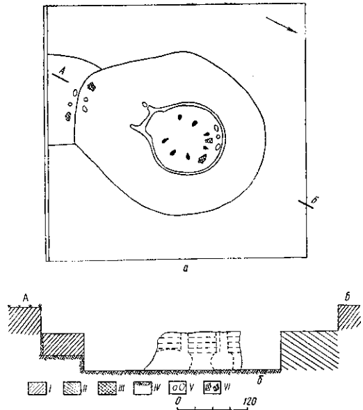
Рис. 3. Гончарне горно з поселення Хлопків I. План (а) та розріз (б):
