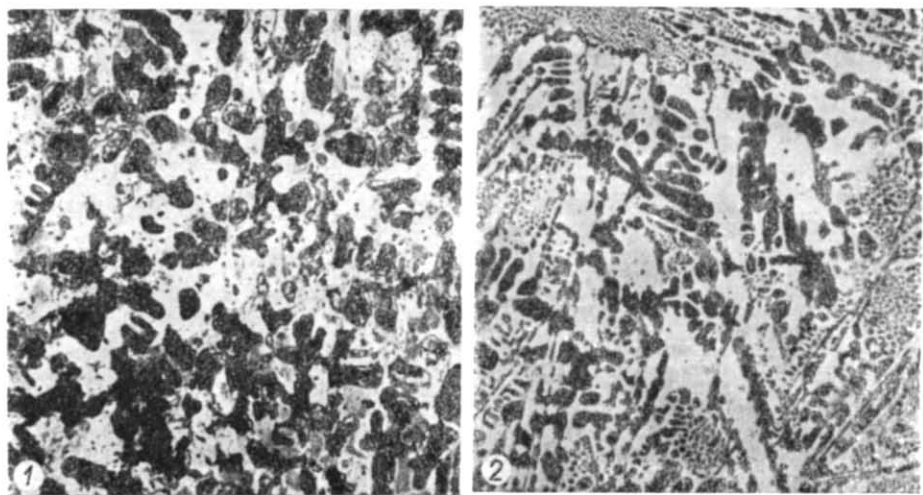
Рис. 4. Мікροструктура зразків \times 160 : 1 — зразок № 3, 2 — зразок № 4.
