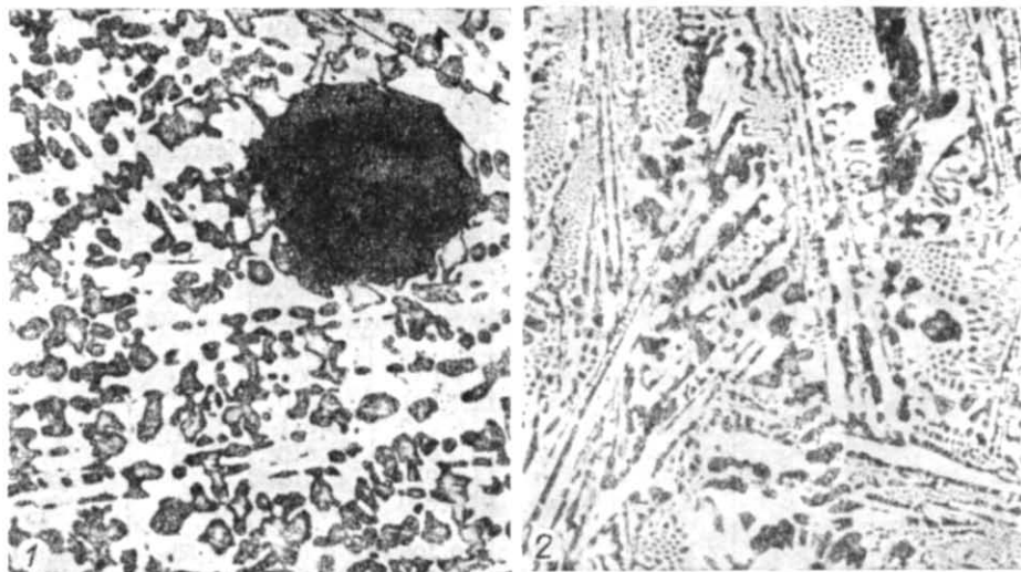
Рис. 3. Мікροструктура зразків \times 160 : 1 — зразок № 1; 2 — зразок № 2.
