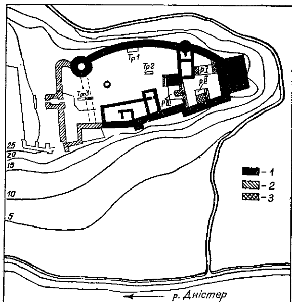
Рис. 1. План кам'яної фортеці в Хотині: 1 — стіни XV ст.; 2 — стіни XVI ст.; 3 — фундаменти XV ст. (відкрито під час розкопок).
