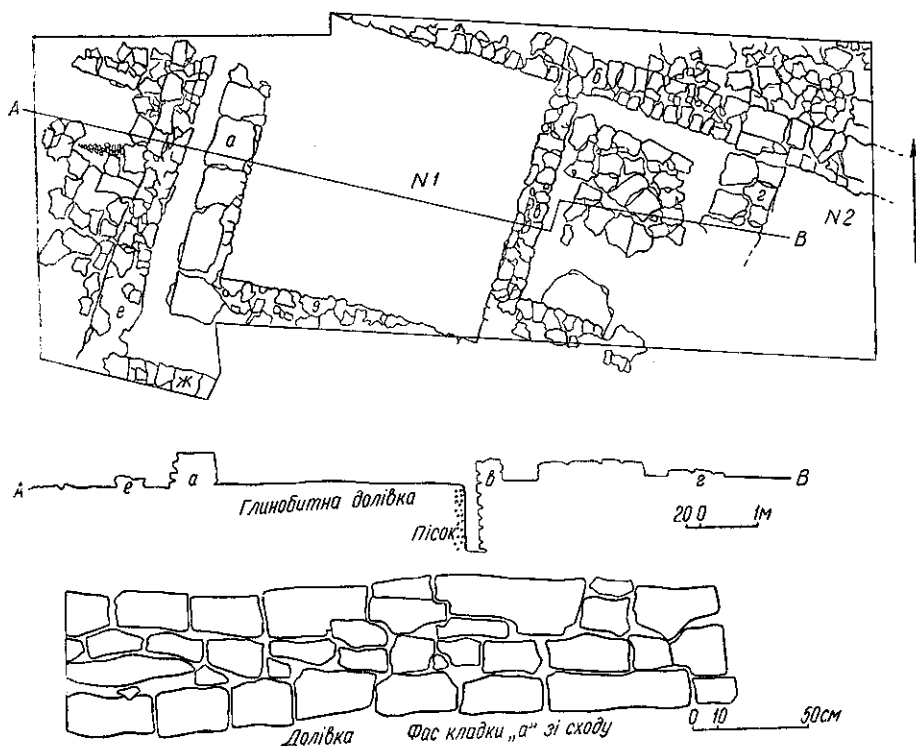
Рис. 1. План розкопаної ділянки.
