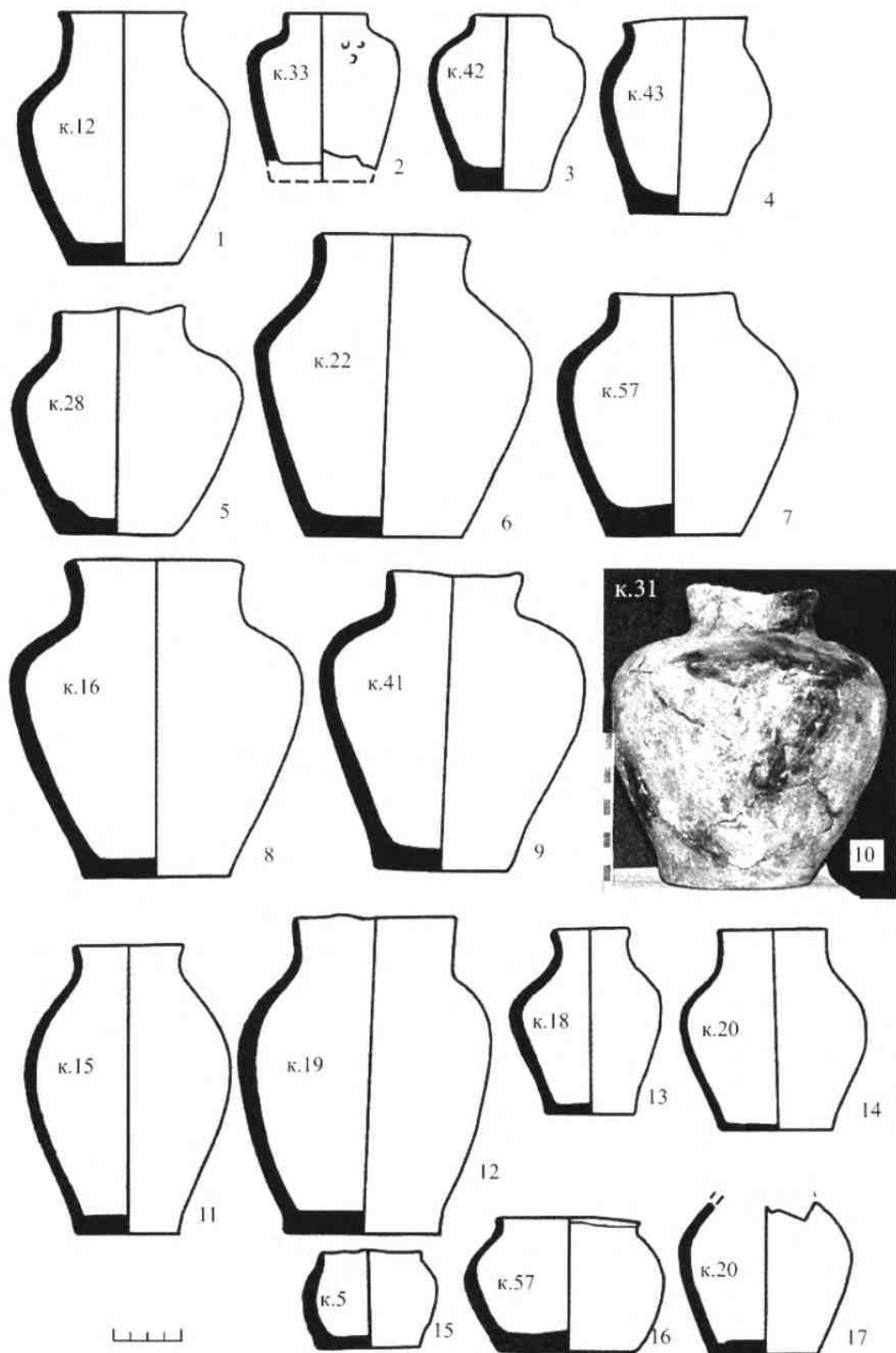
Рис. 7. Салтоидные горшки II Белогорского могильника: 1-10 – тип 7; 11-14 – тип 8; 15-17 – тип 9. Fig. 7. Saltov-like pots from the II nd Belogorsk burial ground: 1-10 – type 7; 11-14 – type 8; 15-17 – type 9
