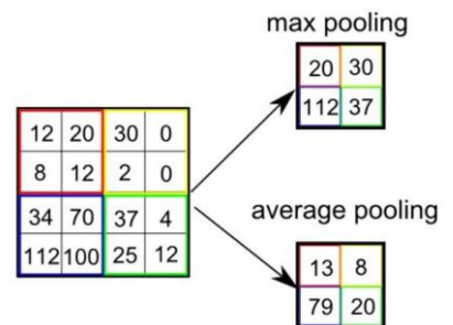
FIG. 5. Pooling layer
